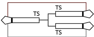
SC7010-□M
